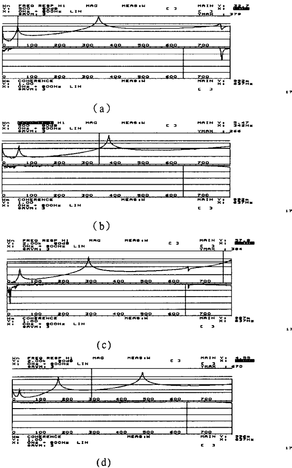
圖七、材料的 FRF 與 Coherence 比較圖 (a) Ti-6Al-4V 材料 (b) 17-4PH 材料 (c) 304SS 材料 (d) FeAlMnC 合金材料
