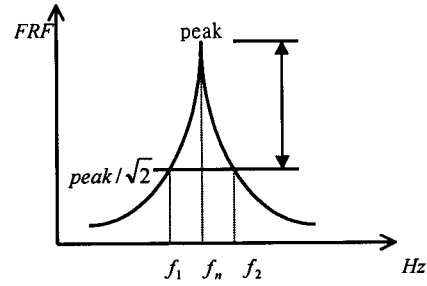
圖二、半能量點之示意圖
