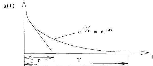
圖三、Exponential 加權函數式意圖
