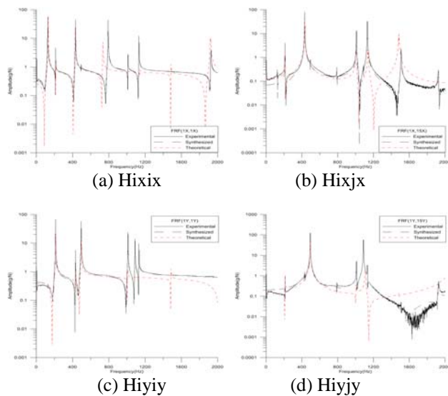
圖 7 實驗與理論頻率響應函數之比較
