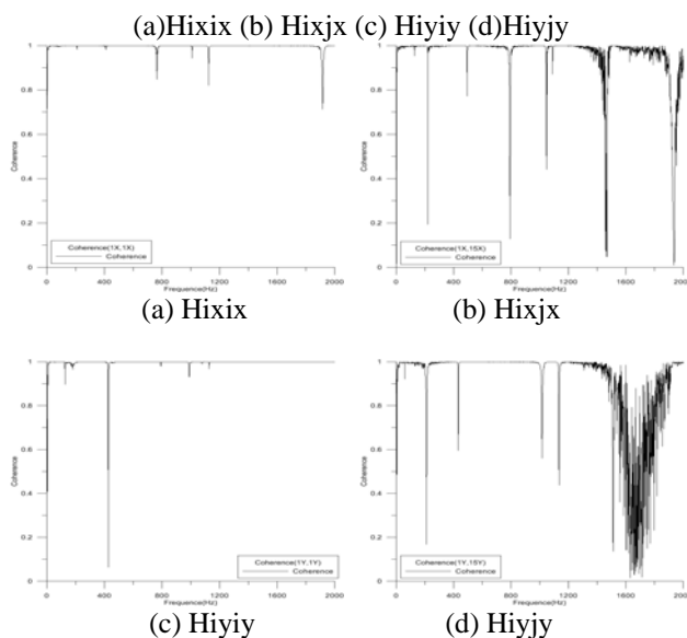
圖 8 關連性函數圖形(a)Hixix (b) Hixjx (c) Hiyiy (d)Hiyjy
