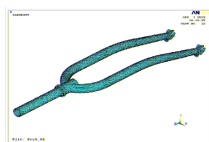
圖 4 前叉有限元素模型
