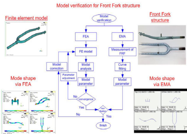
圖 1 模型驗證流程圖
