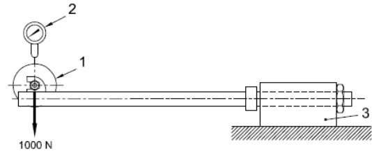
圖 9 EN14764 前叉彎曲試驗規範示意圖
