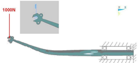
圖 10 前叉彎曲試驗之數學模型圖
