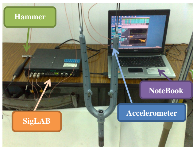
圖 5 實驗架構圖
