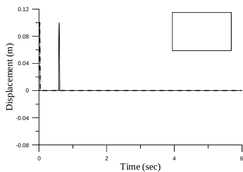
圖 6 前、後輪胎之時間響應 V=5(\text{km/hr})
