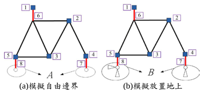
圖 3 模態分析之有限元素模型示意圖
