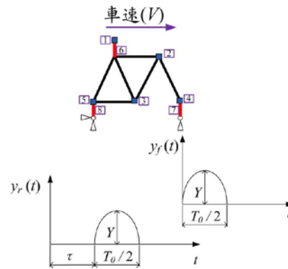
圖 5 行駛於凸起路面狀況示意圖
