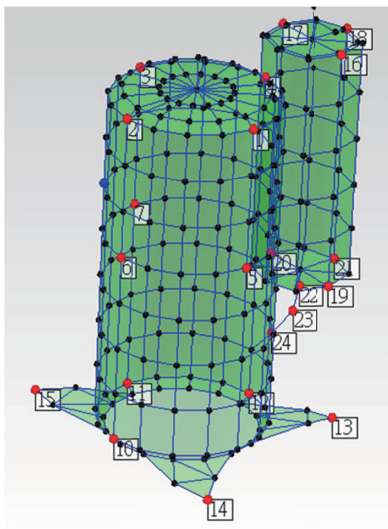
圖 2 壓縮機自由邊界 EMA 布點規劃
