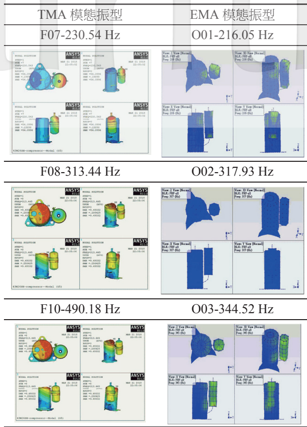
圖 5 壓縮機自由邊界物理意義比對表
