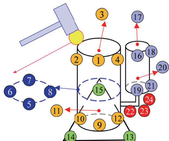
圖 7 壓縮機腳墊邊界 EMA 布點規劃
