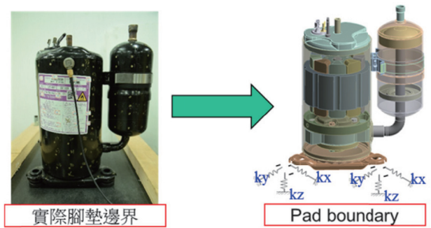
圖 8 壓縮機腳墊邊界實體轉換有限元素模型 註：本文彩色圖，請至電子期刊瀏覽。 http://dx.doi.org/10.6282/JASV
