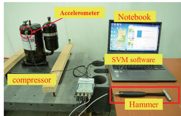
圖 6 壓縮機腳墊邊界實驗儀器與量測圖
