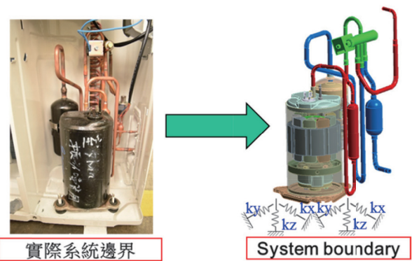
圖 10 壓縮機空調邊界實體轉換有限元素模型 註：本文彩色圖，請至電子期刊瀏覽。 http://dx.doi.org/10.6282/JASV
