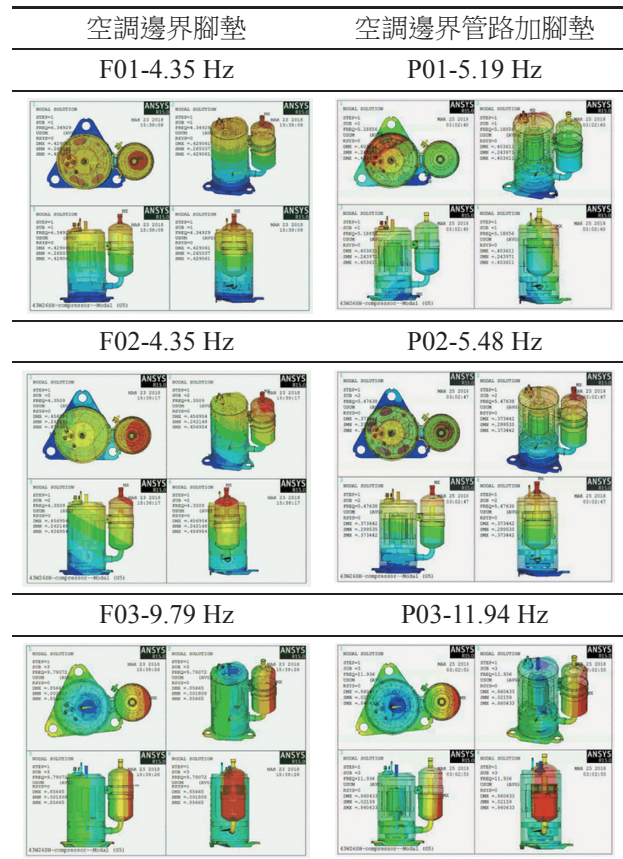
圖 11 空調邊界腳墊與管路加腳墊模態參數物理意義比對表
