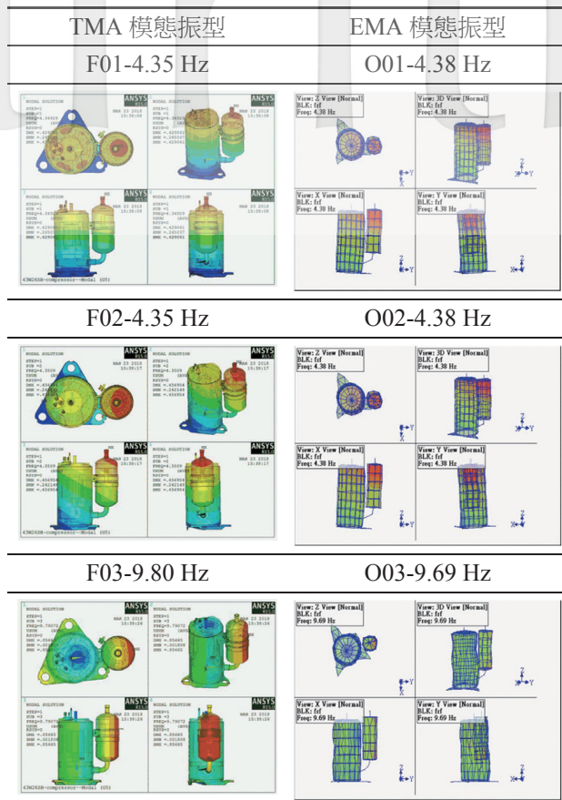
圖 9 腳墊邊界理論與實驗模態參數物理意義比對表 註：本文彩色圖，請至電子期刊瀏覽。 http://dx.doi.org/10.6282/JASV
