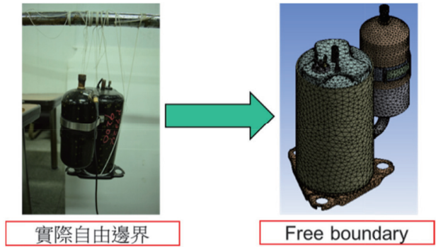
圖 4 壓縮機自由邊界實體轉換有限元素模型 註：本文彩色圖，請至電子期刊瀏覽。 http://dx.doi.org/10.6282/JASV
