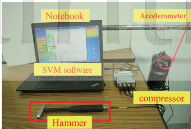
圖 1 壓縮機自由邊界實驗儀器與量測圖
