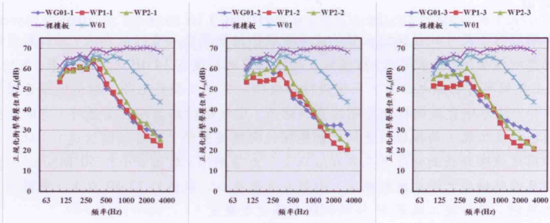
圖 3 木質地板與不同厚度緩衝材之浮式構造樓板正規化衝擊聲壓位準 L_n
