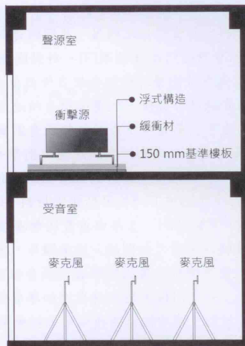
圖 1 本研究浮式地板樓板衝擊音隔音性能量測示意圖
