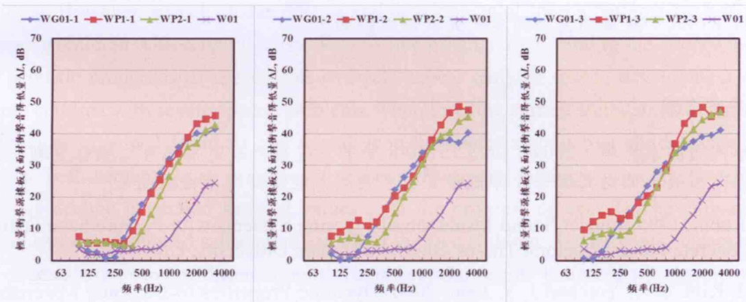
圖 4 木質地板與不同厚度緩衝材之浮式構造樓板衝擊聲壓位準減低量 \Delta L
