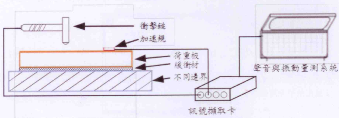
圖 2 浮式地板緩衝材動態剛性量測示意圖[8]
