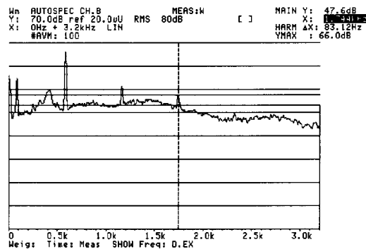
圖 4、運轉中風扇噪音頻譜
